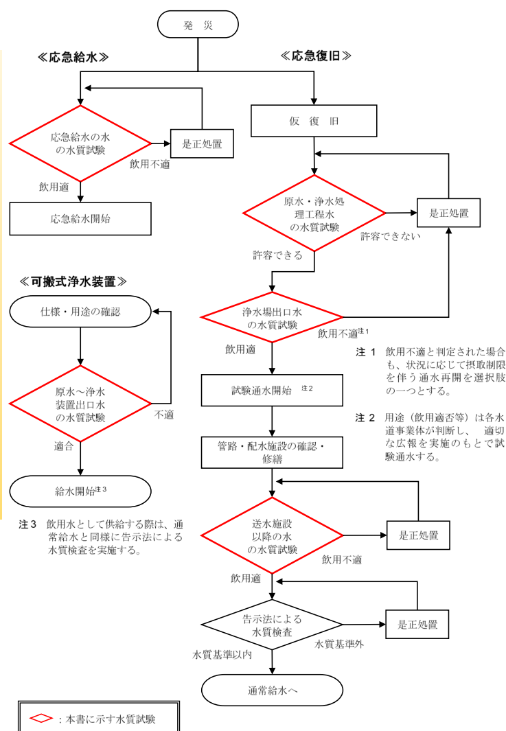
図 発災から通常給水に至る過程の水質試験と判断フロー
